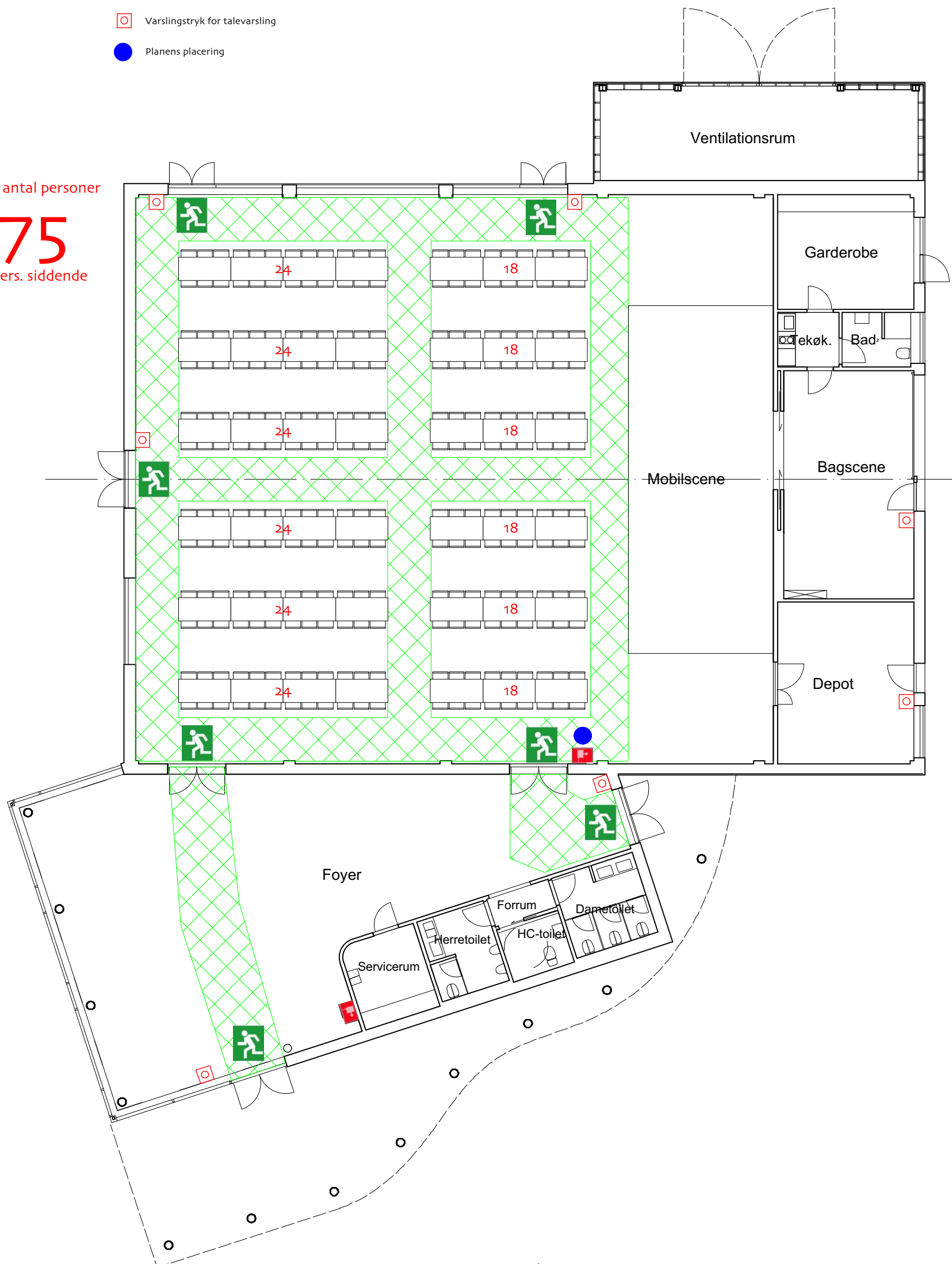
Flugtvejs- og pladsfordelingsplan 4 Skala 1:150 Ollerup Efterskole / Koncerthus
