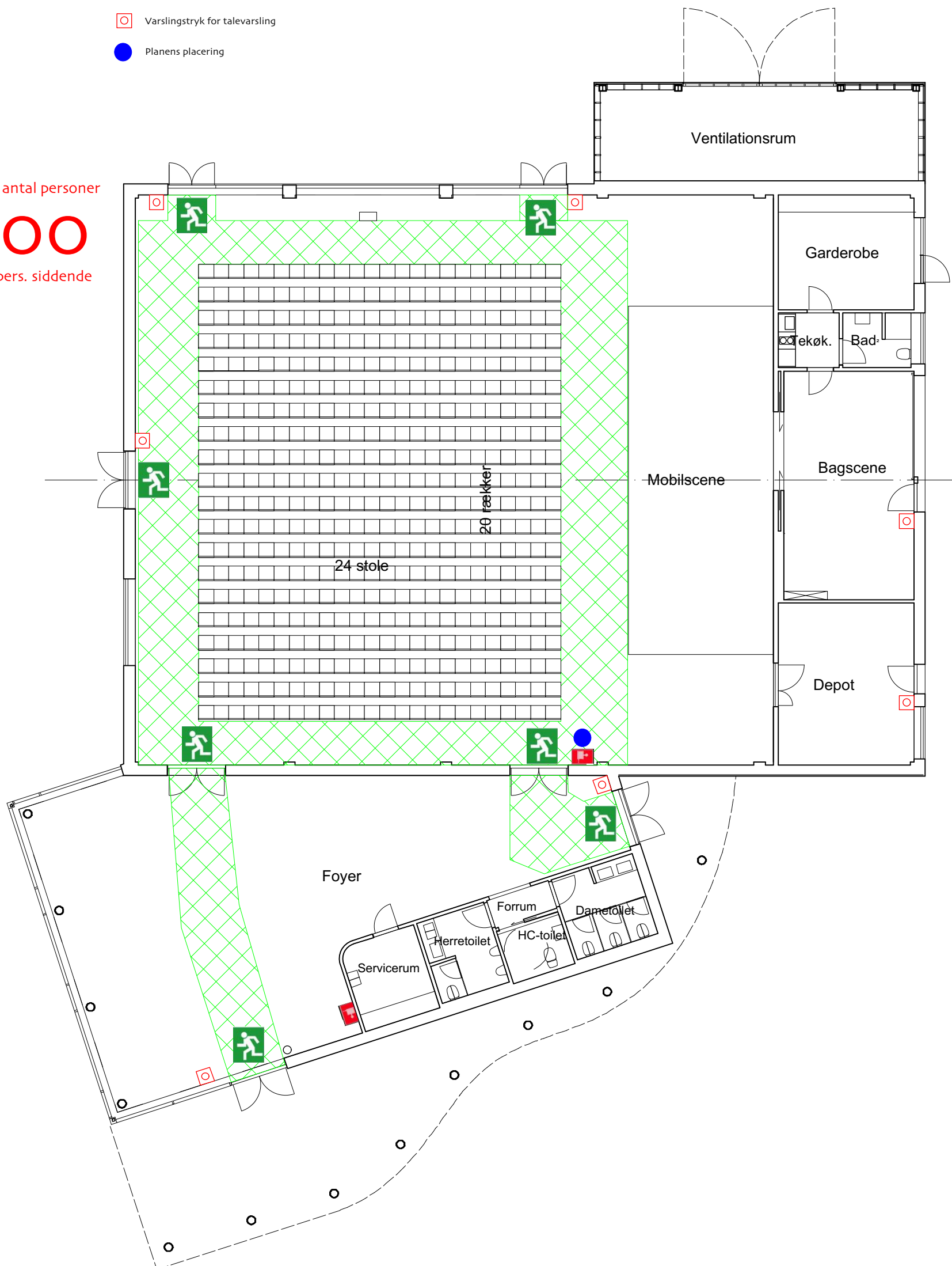
Flugtvejs- og pladsfordelingsplan 2 Skala 1:150 Ollerup Efterskole / Koncerthus
